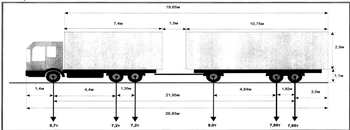
СХЕМА транспортного средства (автопоезда), с использованием которого планируется осуществлять перевозки тяжеловесных и (или) крупногабаритных грузов, с указанием размещения такого груза
